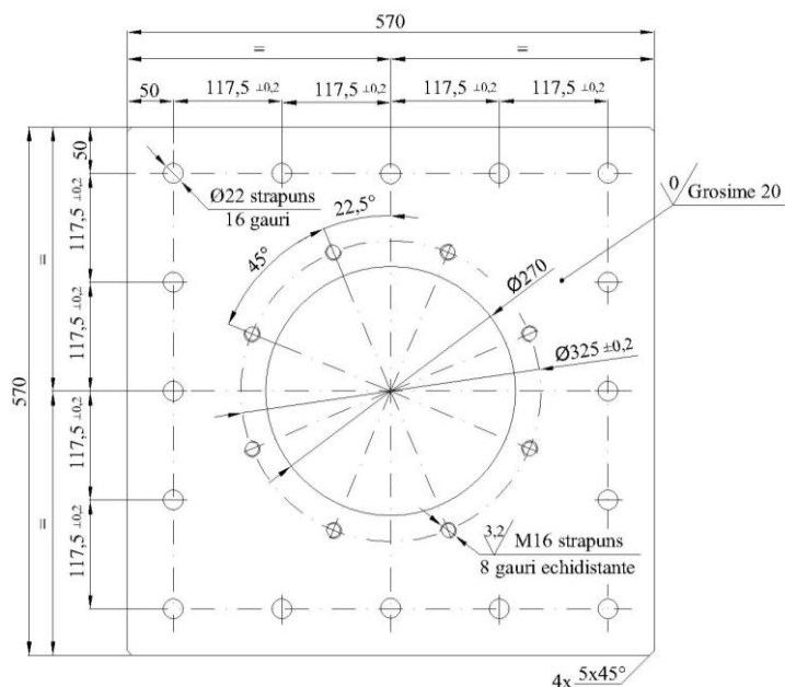
Placa prindere(asigurata de CONFIND)
